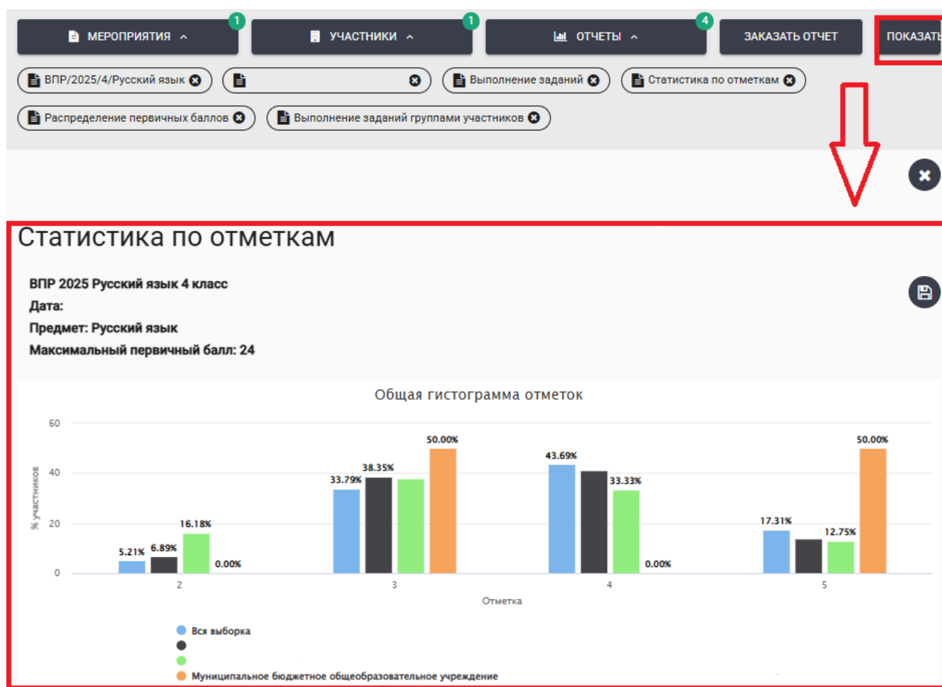
Рисунок 8 – Кнопка «Показать»
