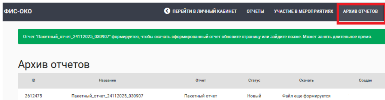
Рисунок 9 – Архив отчетов
