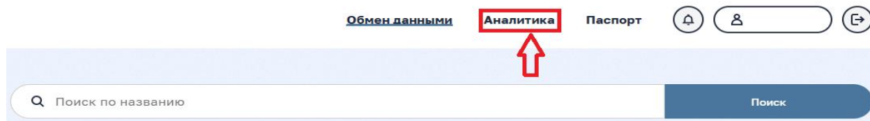
Рисунок 1 – Раздел «Аналитика»
