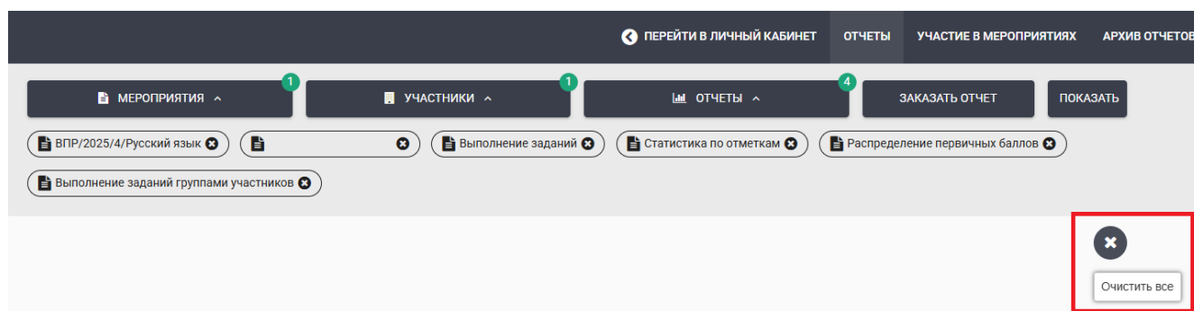
Рисунок 10 – Очистить все
