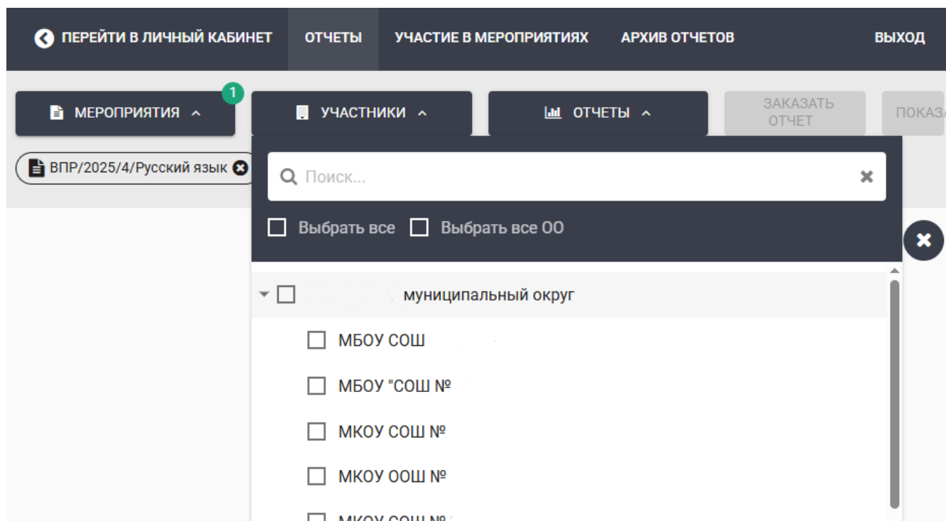
Рисунок 5 – Вкладка «Участники»
