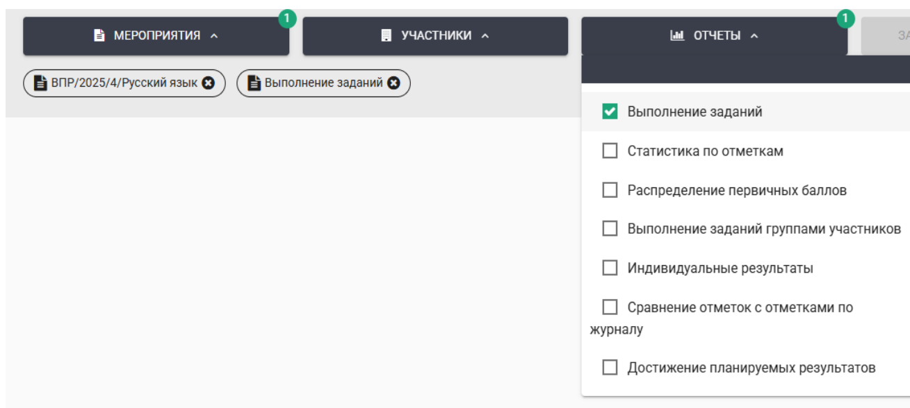
Рисунок 6 – Вкладка «Отчеты»
