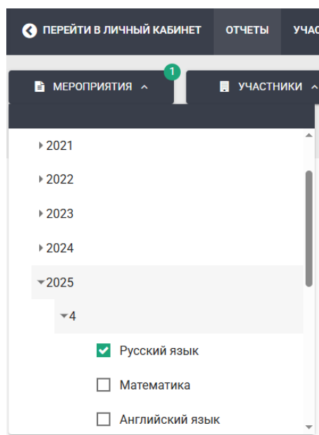
Рисунок 3 – Вкладка «Мероприятия»
